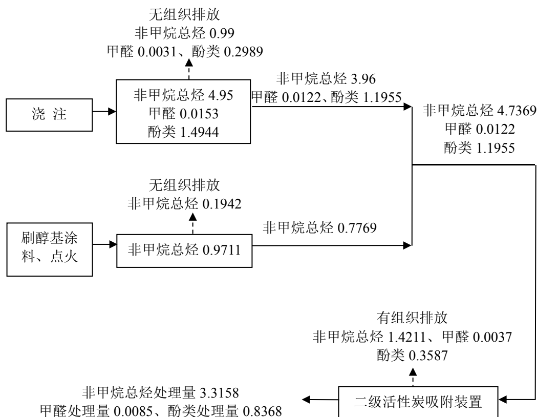
图 2-2 本项目非甲烷总烃、甲醛、酚类平衡图 单位：t/a
