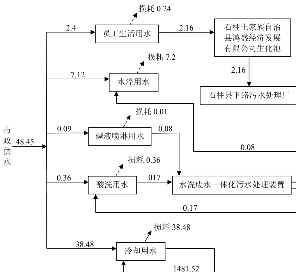
图 2-3 本项目给、排水平衡示意图 单位：m³/d
