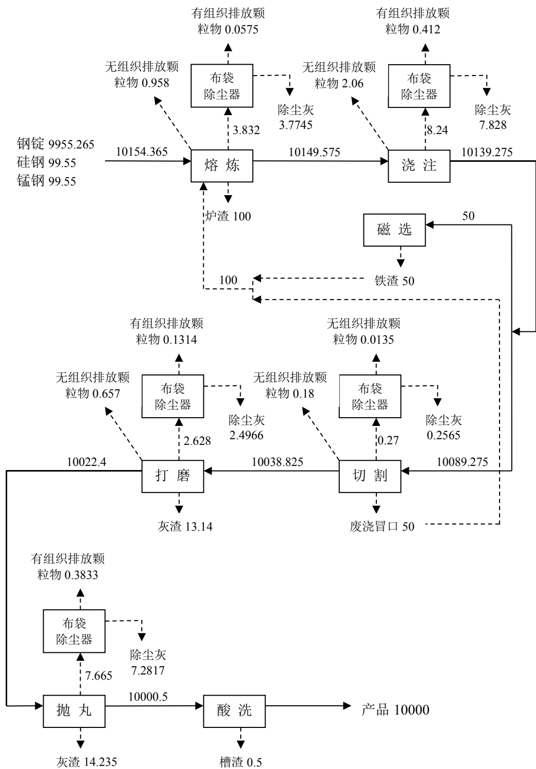
图 2-1 本项目物料平衡图
