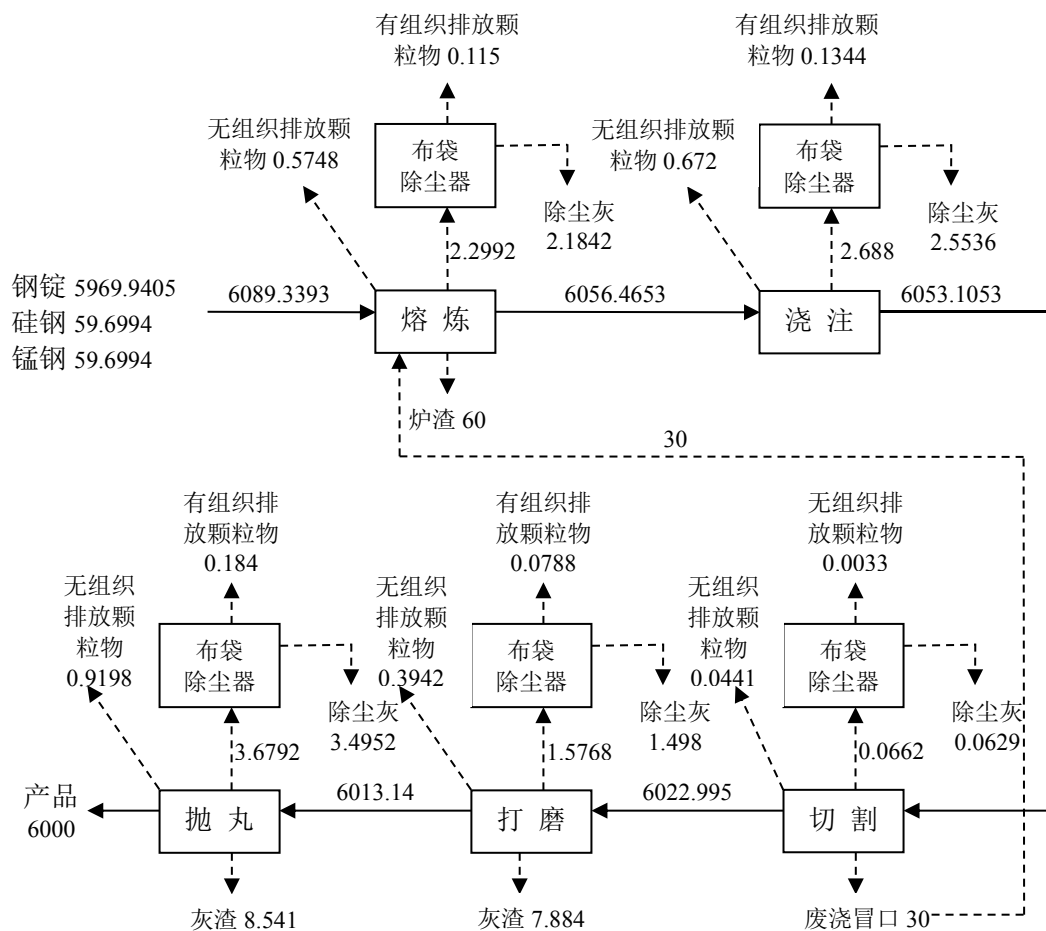
图 2-1 本项目物料平衡图 单位: t/a
