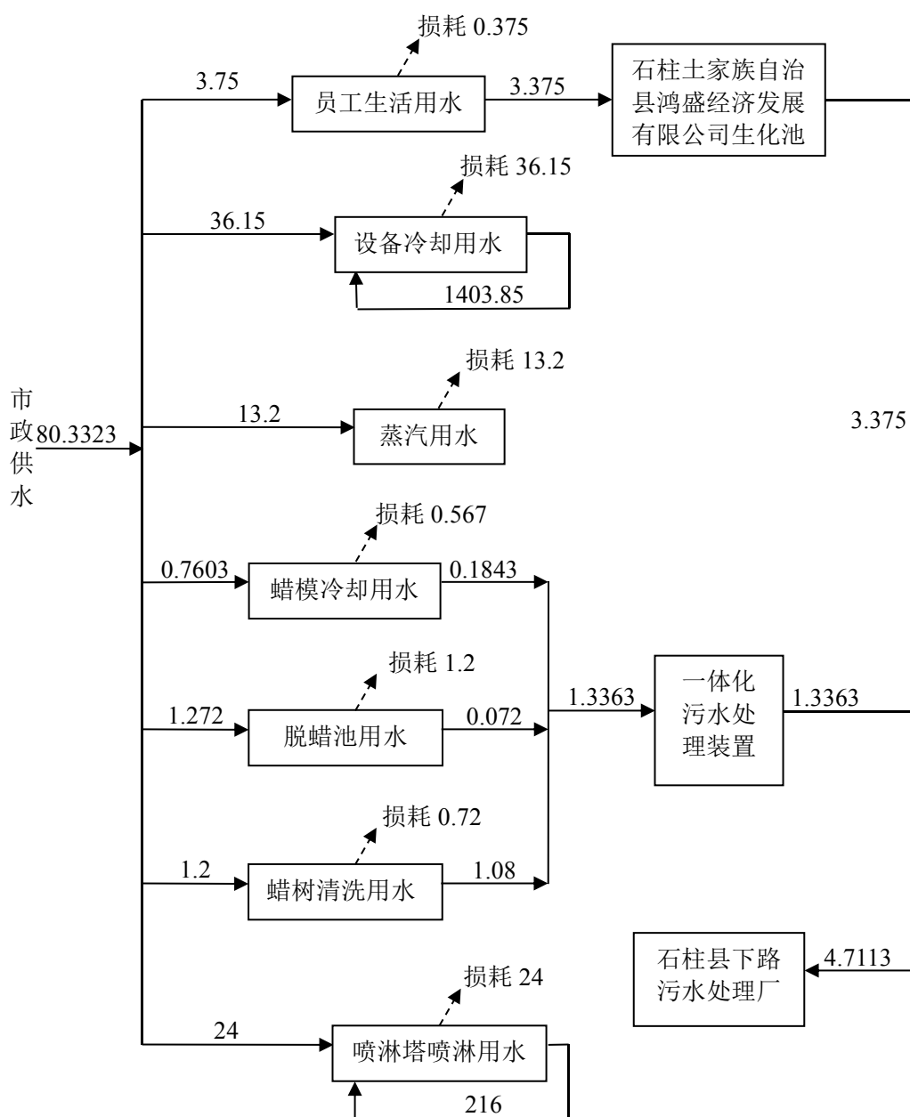
图 2-3 本项目给、排水平衡示意图 单位: m³/d
