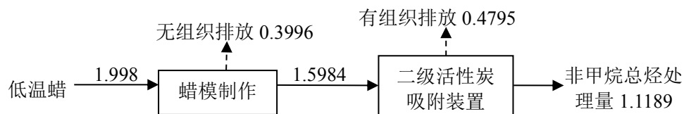
图 2-2 本项目非甲烷总烃平衡图 单位：t/a
