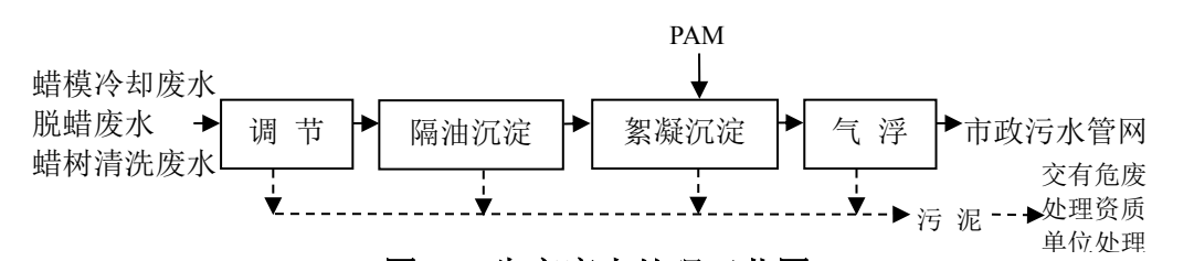
图 4-1 生产废水处理工艺图
